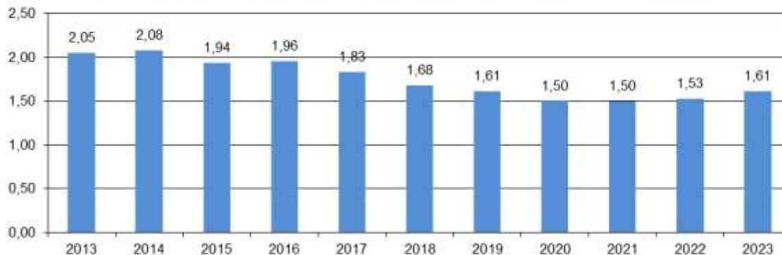
Потребление теплоэнергии на 1 тонну товарной продукции, Гкал/тонна
